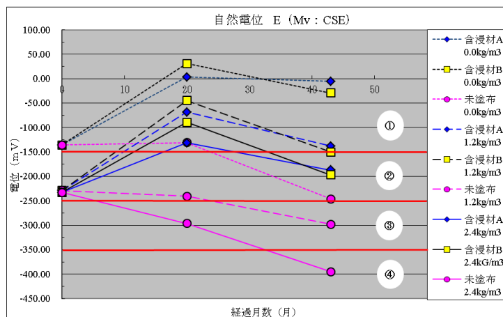
図3 自然電位
