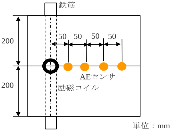
図 2 計測概要
