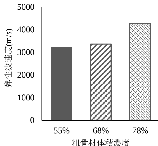
図 4 弾性波速度
