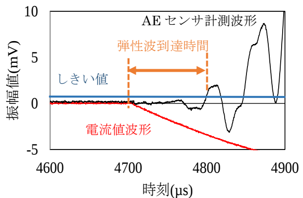
図 3 弾性波到達時間の算出方法
