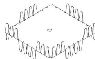
図-1 緊結金具
