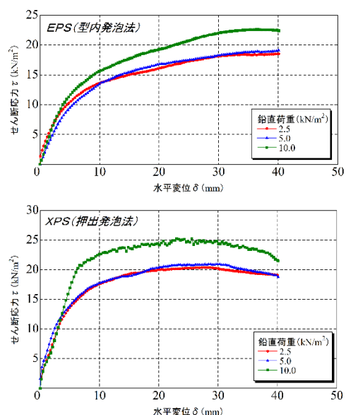
図-3 新金具のせん断応力と水平変位の関係
