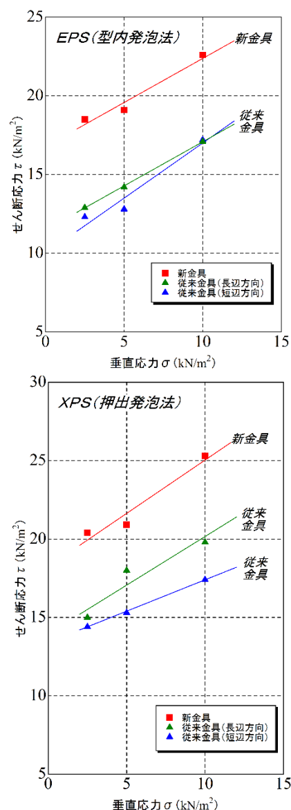
図-4 せん断応力と垂直応力の関係
