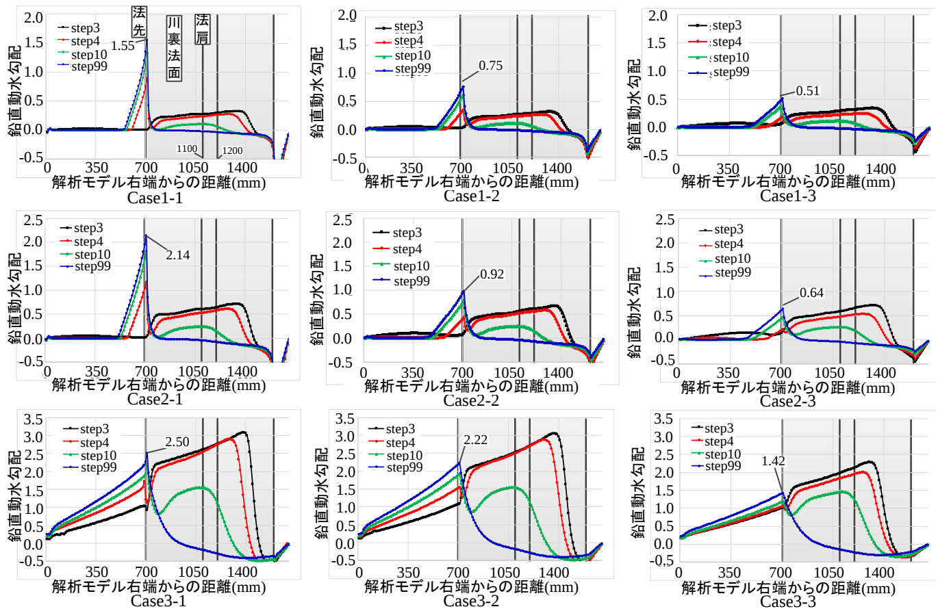
図2 鉛直動水勾配の分布の推移
