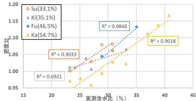
図-5 実測含水比と密度比の関係(変数: 液性限界)
