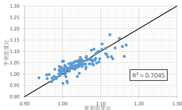
図-7 実測密度比と予測密度比の関係
