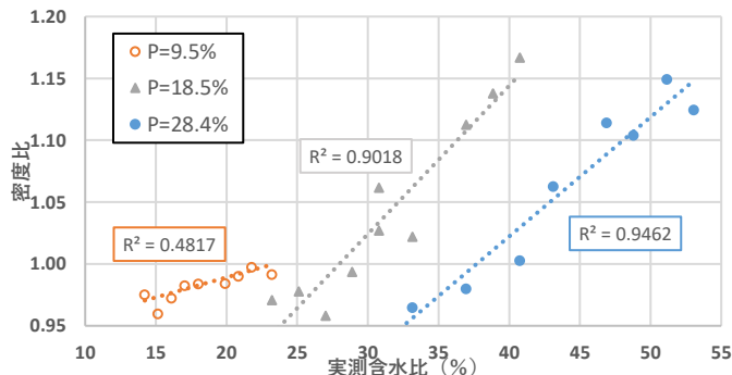
図-4 実測含水比と密度比の関係(変数: 細粒分含有率)
