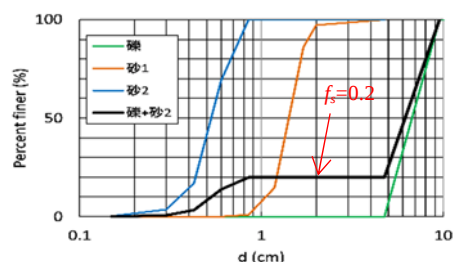
図-1 使用砂礫の粒度分布
