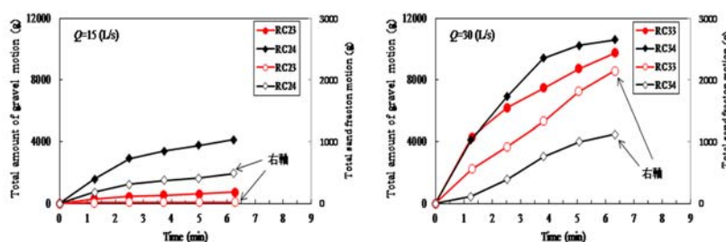
図-5 累積時間と流出土砂量の関係(覆砂量の影響)
