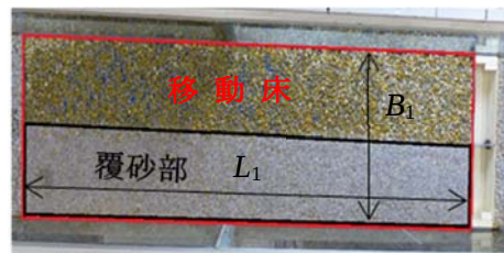
図-2 実験河床
