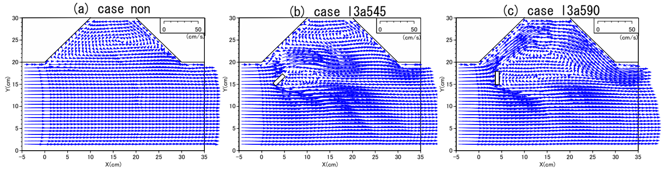
図-2 横断面における時間平均流速ベクトル(台形断面)
