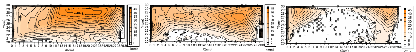
図-5 各ケースの凹部内における土砂堆積形状(8号砂)
