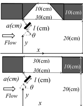
図-1 模型配置図
