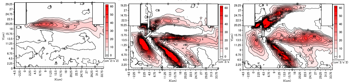
図-4 横断面におけるレイノルズ応力図(z=1.5cm)
