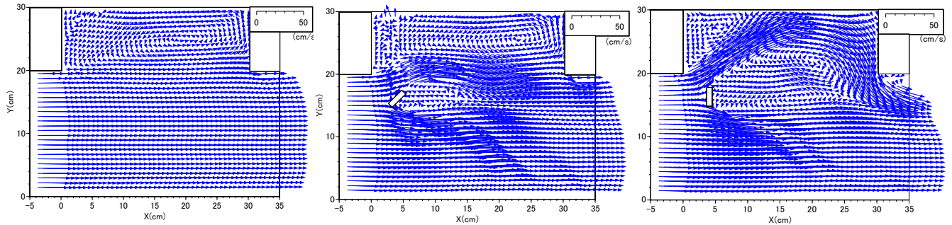
図-3 横断面における時間平均流速ベクトル(長方形断面)
