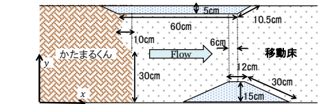
図-3 樹脂固化層Aと水制位置の関係(case1)
