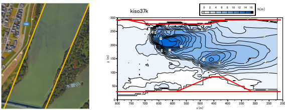
図-1 現地写真 図-2 ADCPによる河床高計測結果 (木曽川上流河川事務所提供)
