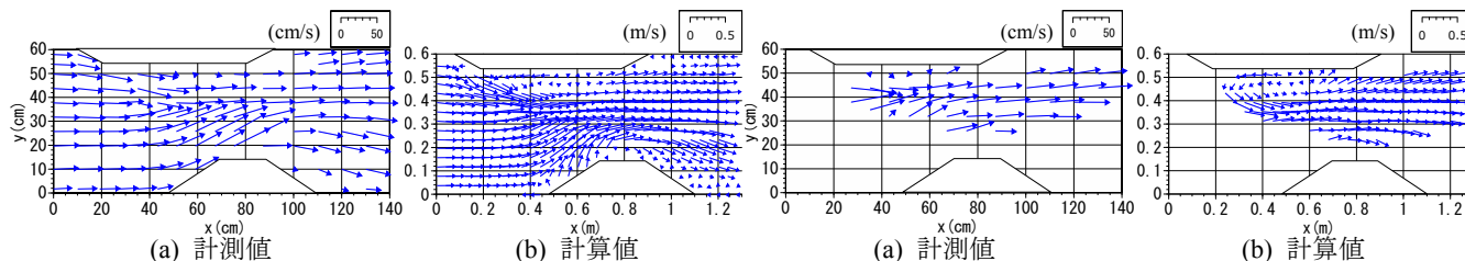
図-6 流速計測結果 (z=1cm)
