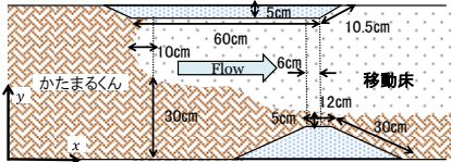
図-4 樹脂固化層Bと水制位置の関係(case2)
