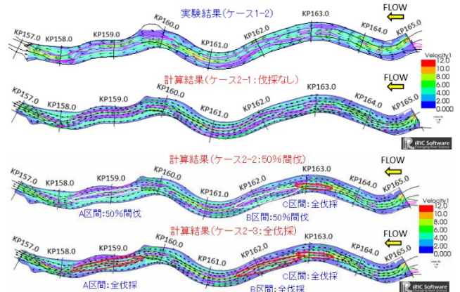
図-6 実験と計算の流速コンター図
