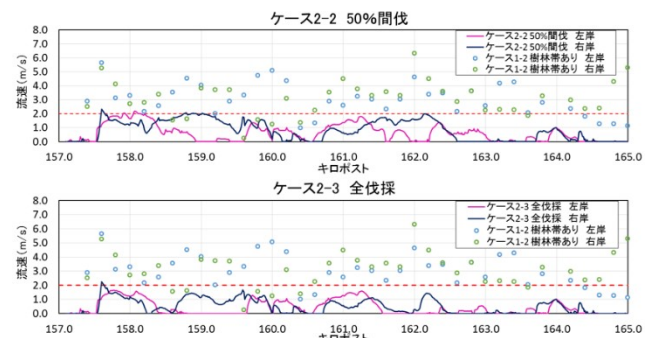
図-7 堤防沿いの流速の比較
