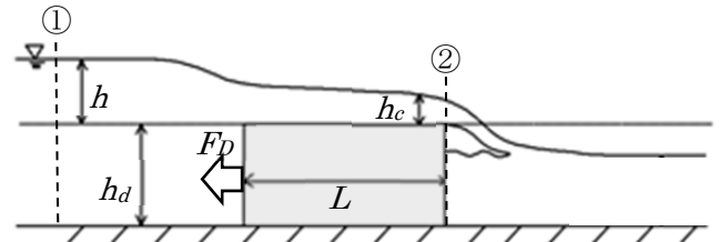
図-1 広頂堰を越える流れの模式図
