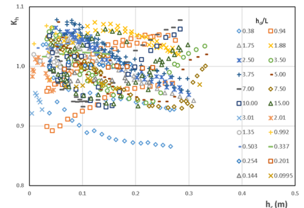
図-6 越流水深評価式の適用結果
