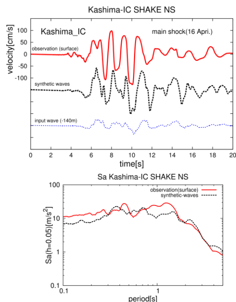
(a)本震時の速度記録と加速度応答スペクトル
