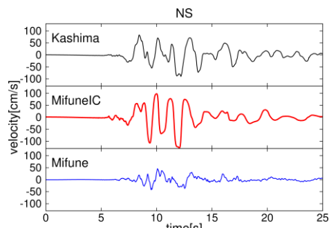
図 1:熊本地震本震における速度波形(南北成分)の比較
