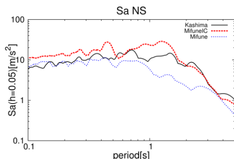
図 2:熊本地震本震における加速度応答スペクトル(南北成分)の比較
