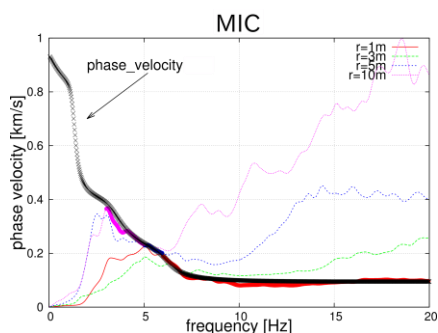
図 4:推定した Rayleigh 波基本モードの位相速度
