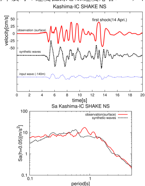
(b)前震時の速度記録と加速度応答スペクトル
