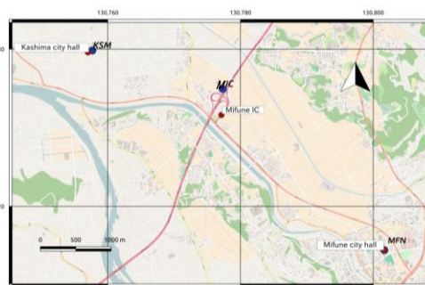
図 3:地震計の位置と微動アレー観測の実施地点
