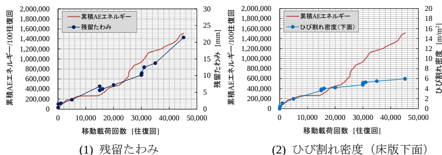
図-2 累積 AE エネルギーと移動載荷回数の関係
