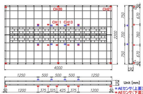
図-1 AE センサの設置位置
