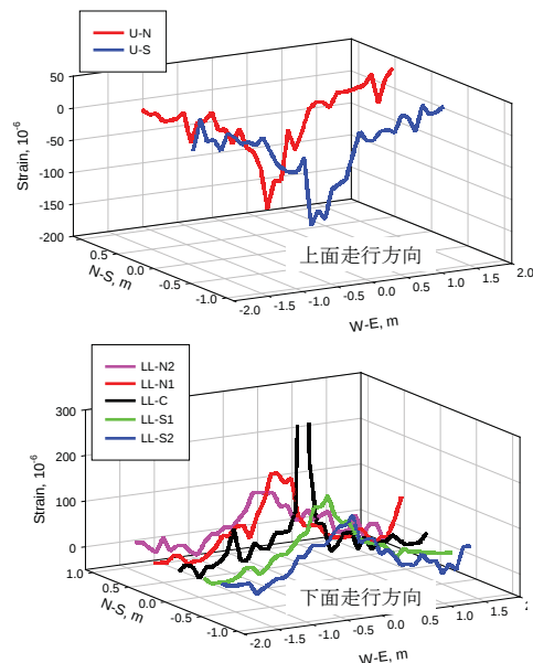
図-2 ひずみ分布例
