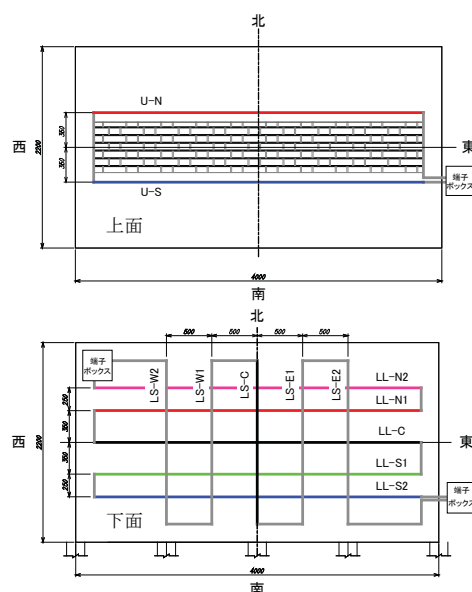
図-1 光ファイバーセンサ配置
