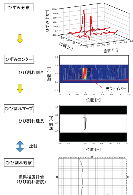
図-3 評価指標の処理フロー
