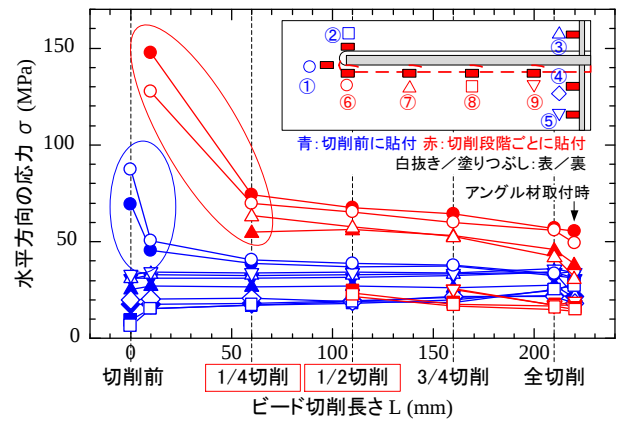
図-3 切削長さ L と応力 \sigma の関係 (試験部 A)
