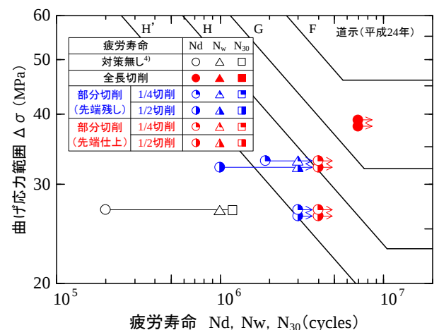
図-4 各試験部の疲労寿命
