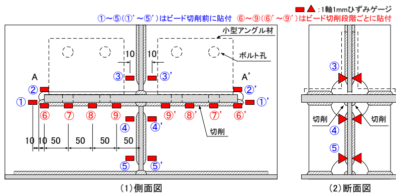
図-2 試験体 A 貫通部の拡大図
