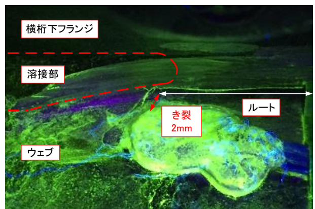
写真-2 試験部 B' のき裂発見状況 (N=190 万回)
