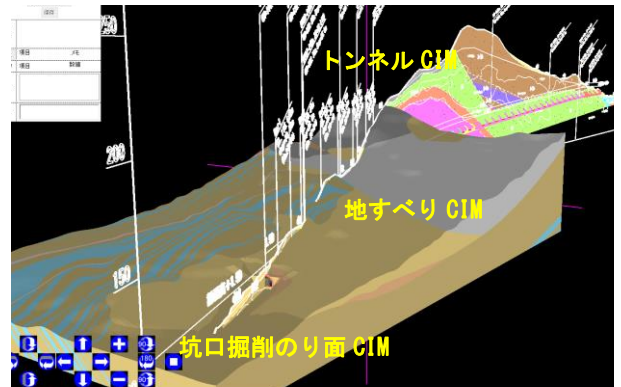
図-1 トンネルにおけるCIM表示例
