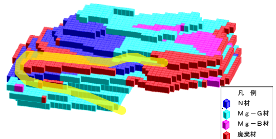
図-3 3次元GIS賦存量管理モデル
