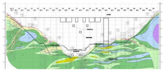
図-2 ダムにおける地質縦断面図の例
