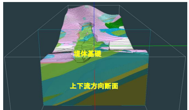
図-5 任意の位置における断面図表示例
