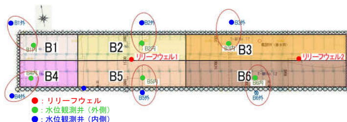
図-1 リリーフウェルと観測井の配置図
