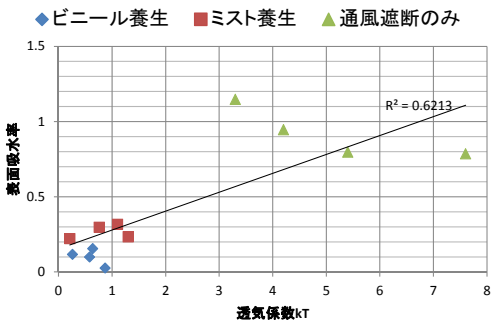
図-5 表面吸水率と透気係数の関係
