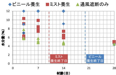
図-2 水分計測定結果
