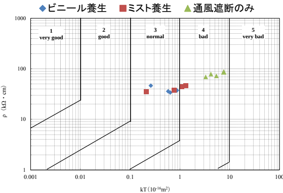
図-4 透気試験評価
