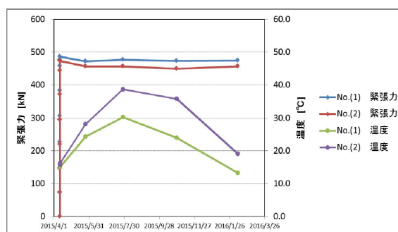
図-3 EMセンサー緊張力測定結果
