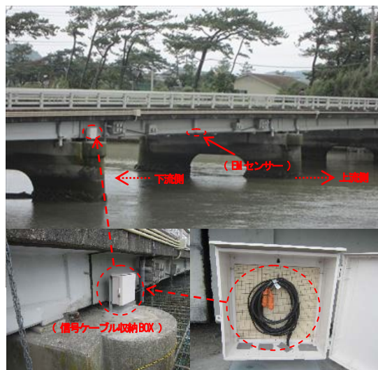
写真-4 館山大橋
