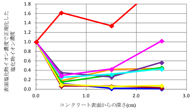
図-3 張出部下面の塩化物イオン濃度の関係
