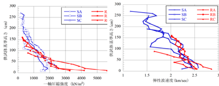
図-2 弾性波速度と供試体高さの関係
