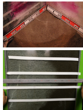
図-8 クラックの状況
