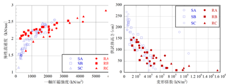
図-3 一軸圧縮強度と弾性波速度の関係
