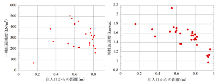
図-5 一軸圧縮強度と注入距離の関係
