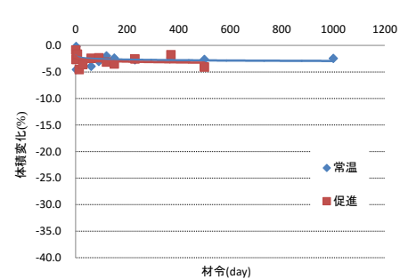
図-3 活性シリカコロイドホモゲル体積変化
