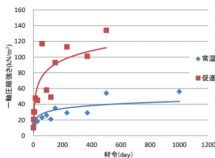
図-2 活性シリカコロイドホモゲル強度
