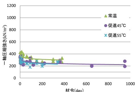
図-4 シリカゾルサンドゲル強度
