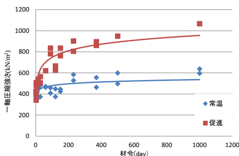
図-1 活性シリカコロイドサンドゲル強度
