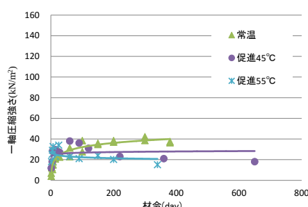
図-5 シリカゾルホモゲル強度
