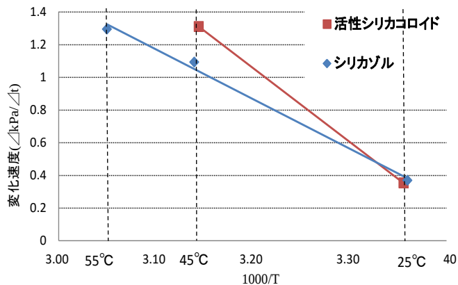
図-7 サンドゲルのアレニウスプロット
