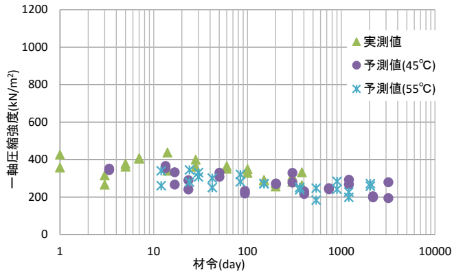
図-9 シリカゾルサンドゲルの予測強度
