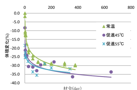
図-6 シリカゾルホモゲル体積変化
