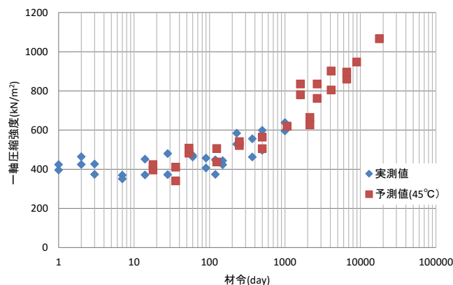
図-8 活性シリカコロイドサンドゲルの予測強度
