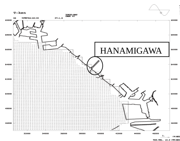
図-7 花見川河口周辺流速分布(下げ潮)
