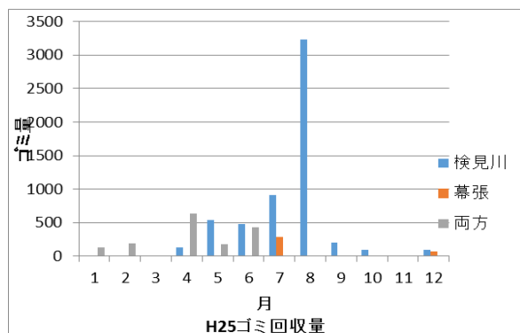
図-4 ゴミ回収量(平成 25 年)
