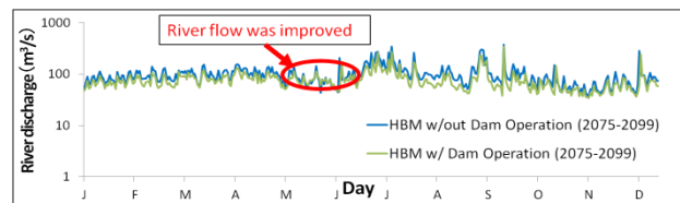
図1 吉野川流域岩津地点の年間日別時系列流量
