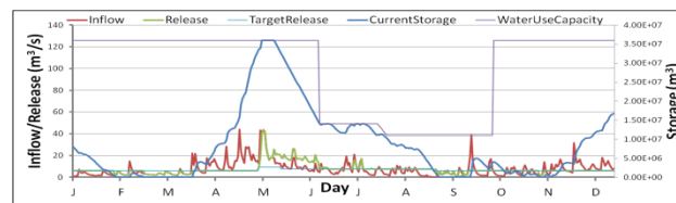
図3 1979年における白川ダムの操作結果例
