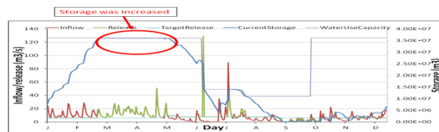
図4 2075年における白川ダムの操作結果例
