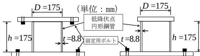
図-1 頭部固定有り(左)・頭部固定無し(右)
