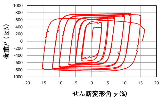
図 - 4 頭部固定有り 履歴曲線
