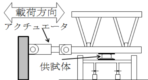
図-2 実験装置概要図
