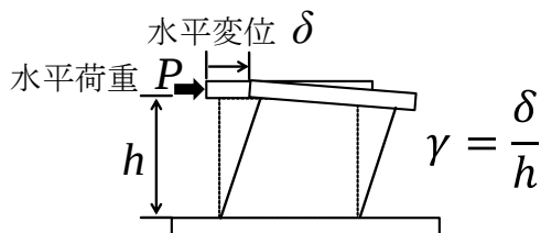
図-3 変形状態の模式図
