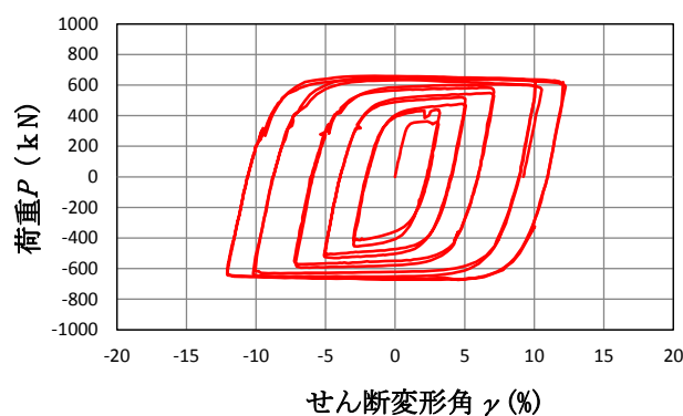
図 - 5 頭部固定無し 履歴曲線
