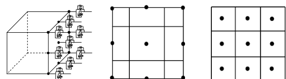
図1 要素表面のばね設置の様子とばね設置点(黒点) (左:ばね設置の様子, 中:従来, 右:提案)
