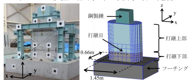
図2 供試体(左)および解析モデル(右)
