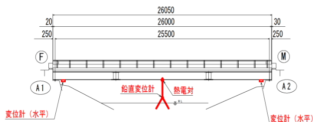
図-1 側面図・計測器設置概要図
