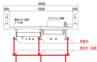
図-3 断面図・計測器設置概要図
