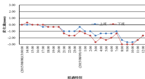
図-6 橋台間の伸縮挙動
