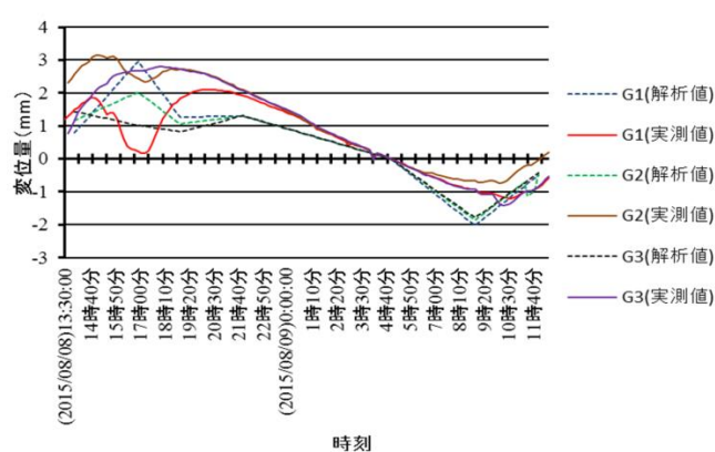
図-7 鉛直変位の実測値と解析値
