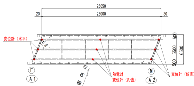
図-2 平面図・計測器設置概要図
