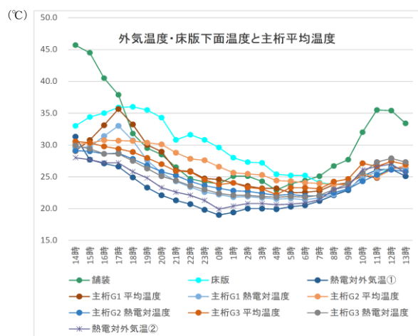
図-5 実橋における温度変化
