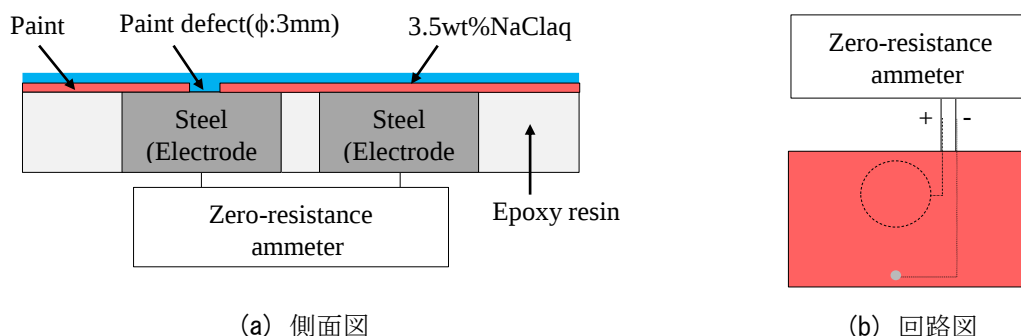
図-1 試験体の概略図
