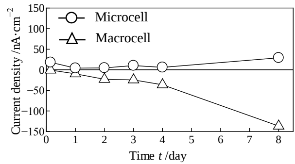
図-3 マクロセル・ミクロセル腐食電流密度
