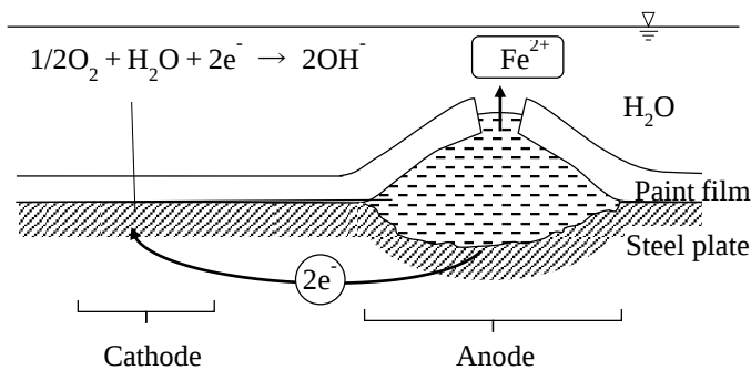
図-4 塗膜傷とその近傍の電氣的短絡の推定図
