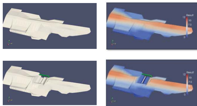
図 2. 3 次元モデル (3 次元 CAD に、相対高さ属性を付加して、掘削による応力解放リスクをカラーコンタで表示)
