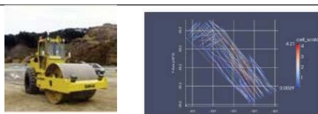
図 3. GPS 搭載重機と転圧軌跡図 (GPS から得られる振動ローラの 3 次元の位置情報からは、盛土の転圧回数の管理により盛土品質の管理を行っている。)
