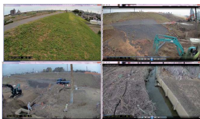
図 6. DB 画面（4 方向映像）（工事空間を 4 方向のカメラで捉えて、工事記録として短時間でタイムラプス映像が確認できる。）
