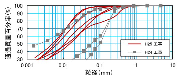
図-3 原料土の粒度分布
