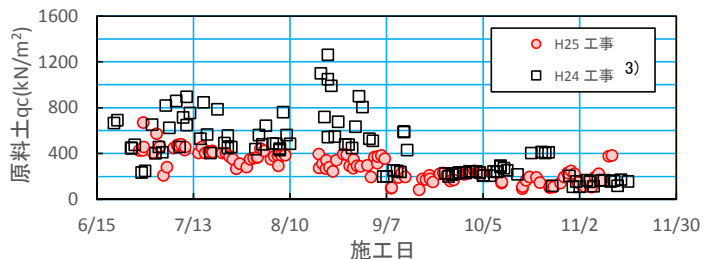
図-2 原料土のコーン指数
