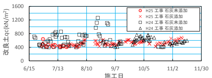
図-4 改良土のコーン指数
