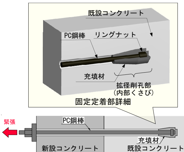
図-1 固定定着構造の概念図
