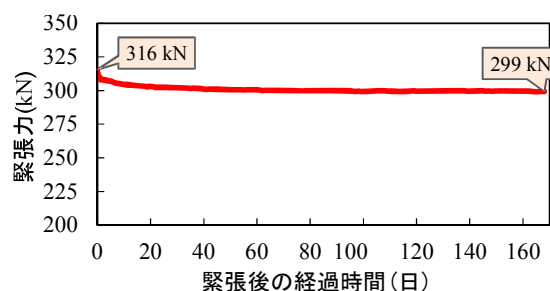
図-5 緊張力の経時変化
