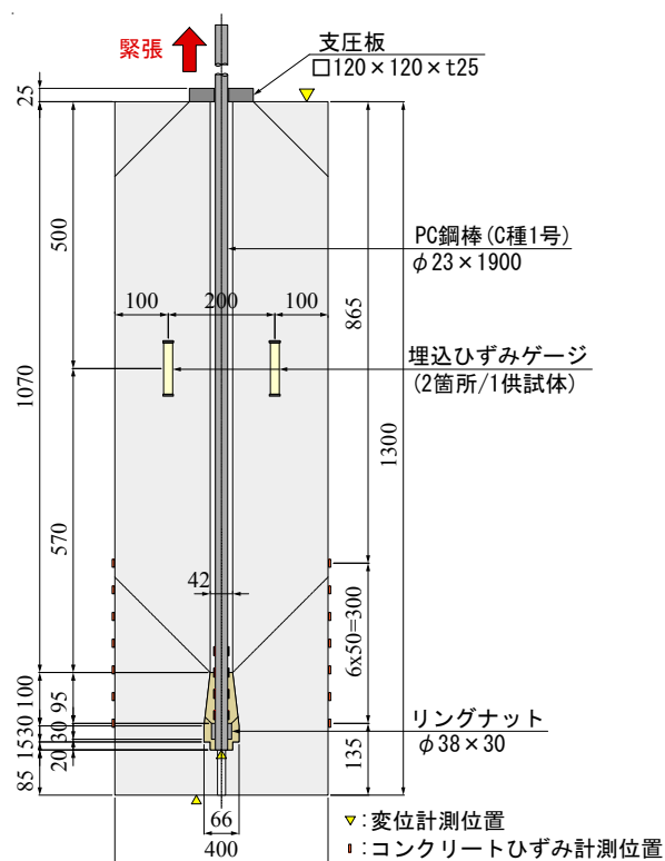
図-2 実験供試体
