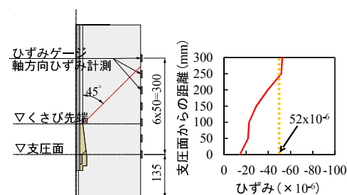
図-4 コンクリート表面の軸方向ひずみ分布 (荷重荷重 350kN 時点)
