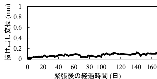
図-6 抜け出し変位の経時変化
