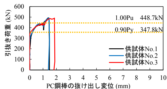
図-3 固定定着部の抜け出し変位
