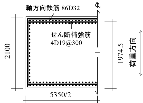
図4 既存不適格の橋脚の断面
