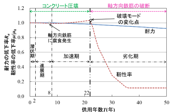
図6 耐力・靱性率の低下率の経年変化
