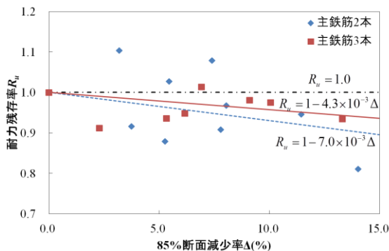
図2 鉄筋断面減少に応じた耐力残存率
