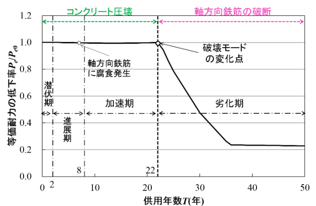
図7 等価耐力の経年変化
