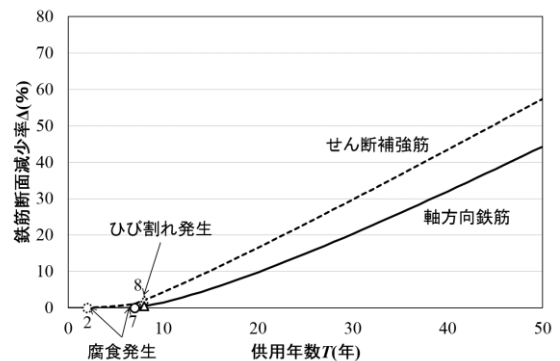
図5 鉄筋断面減少率の経年変化
