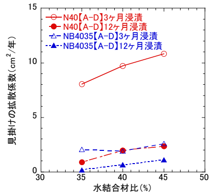
図-2 水結合材比と見掛けの拡散係数の関係
