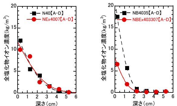
図-4 膨張材添加の影響
