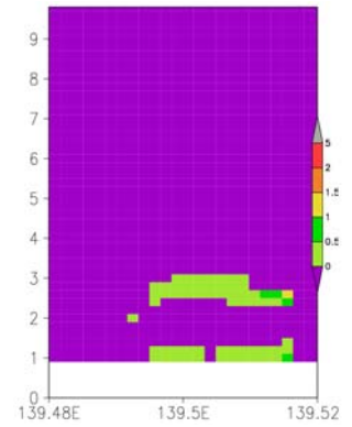
図-3 K_{DP} の鉛直断面図 (2014.06.23 12:40)
