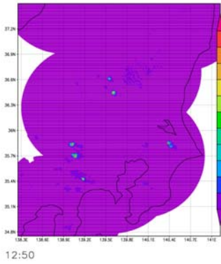
図-1 合成雨量図 (Tokyo 2014.06.23 12:50)
