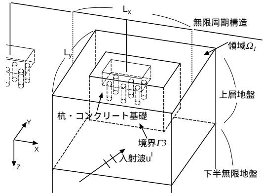
図1 対象とする3次元解析モデルの1ユニット
