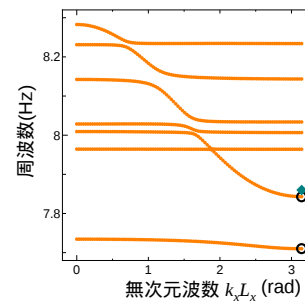
図3 トラス部の分散曲線
