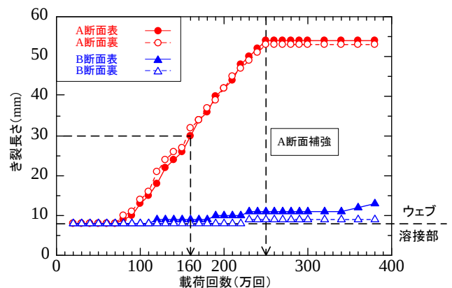
図-3 载荷回数とき裂長さの関係
