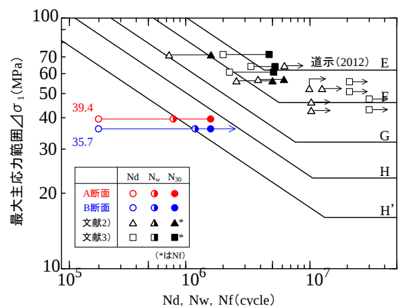
図-4 最大主応力範囲で整理した S-N 線図
