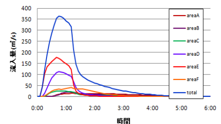
図 7 地下流入量
