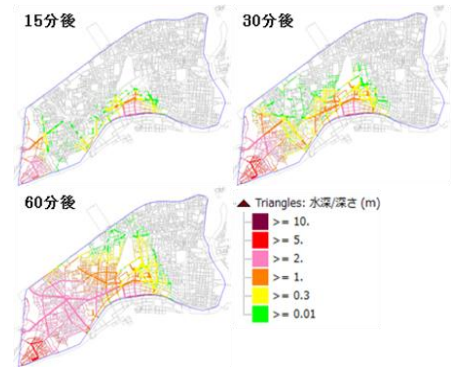
図 3 地下流入を考慮した道路浸水状況
