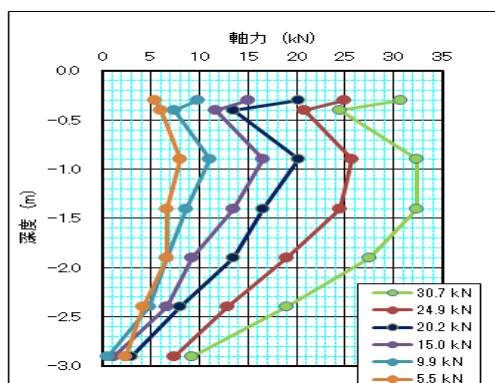
図-4-1 深度-軸力(3m 杭)
