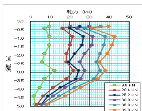
図-4-2 深度-軸力(5m 杭)
