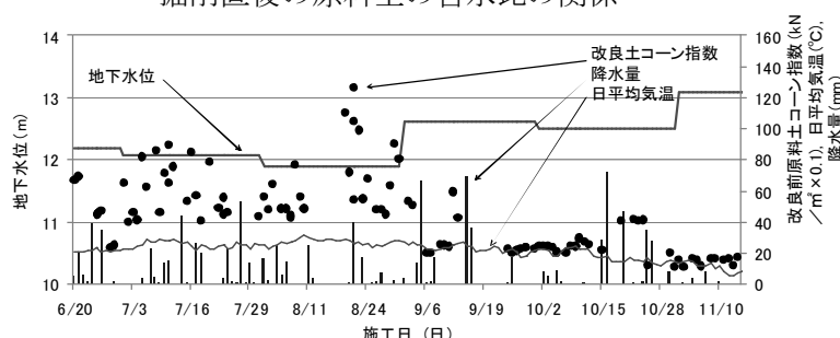
図-3 施工日と降水量と調節地内の地下水位と仮置き改良前の原料土のコーン指数の関係
