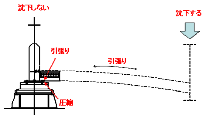
図-3 列車通過時の模式図
