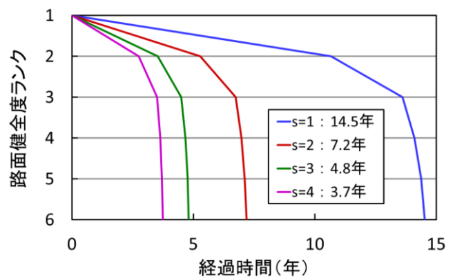
図-2 路面健全度のパフォーマンスカーブ
