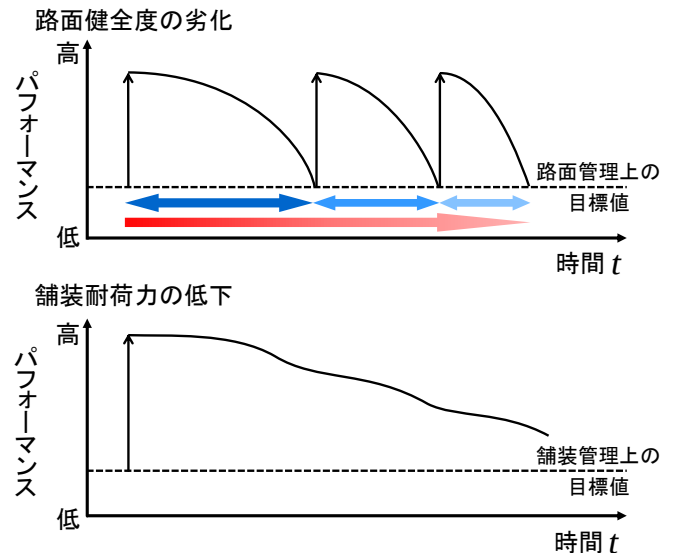
図-1 路面と耐荷力の複合的劣化過程
