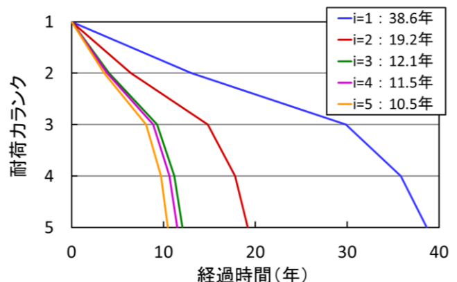
図-3 耐荷力のパフォーマンスカーブ
