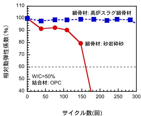
図1 高炉スラグ細骨材が凍結融解抵抗性に及ぼす影響
