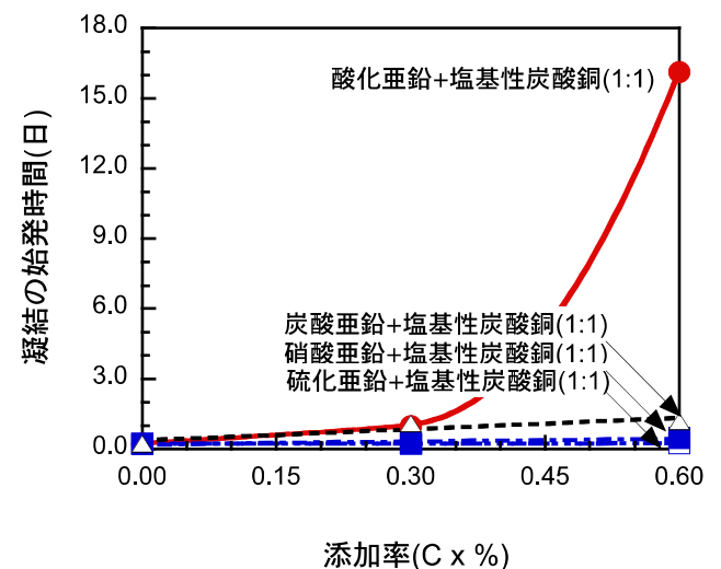
図4 亜鉛化合物と塩基性炭酸銅の混合添加がモルタルの始発時間に及ぼす影響
