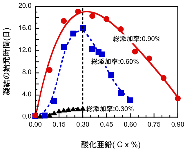
図5 酸化亜鉛と塩基性炭酸銅の混合添加がモルタルの始発時間と終結時間に及ぼす影響
