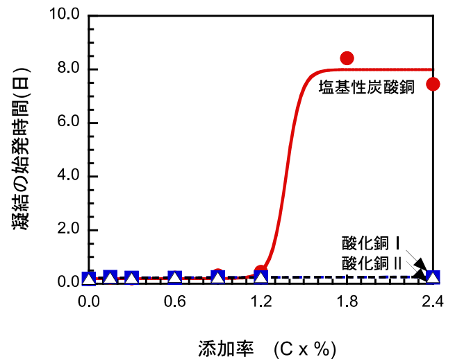
図2 銅化合物がモルタルの凝結時間に及ぼす影響
