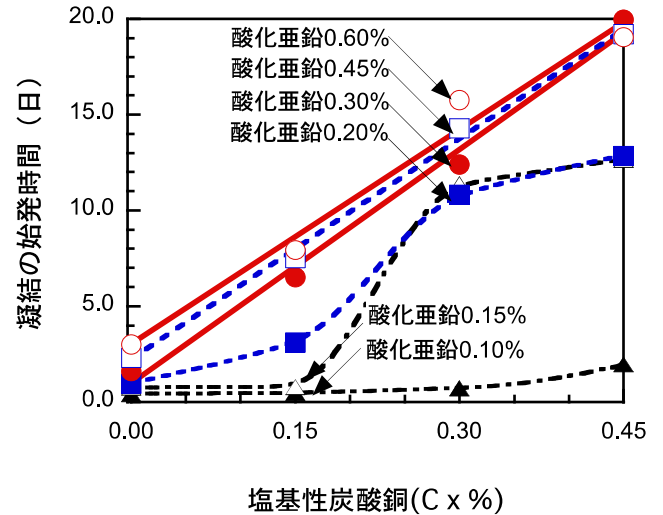
図6 酸化亜鉛と塩基性炭酸銅の混合比率がモルタルの始発時間と終結時間に及ぼす影響
