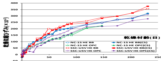
図-2 長さ変化試験(気中のみ)
