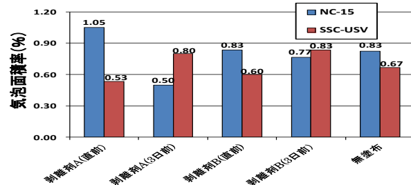
図-4 表面性状評価結果
