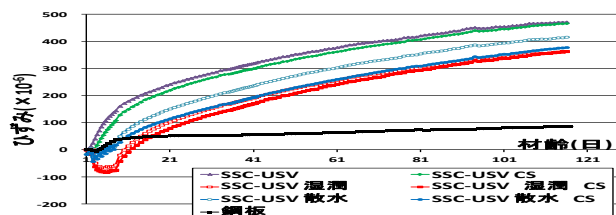
図-3 拘束有の場合の長さ変化試験結果(SSC-USV)
