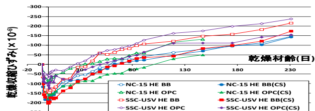
図-1 長さ変化試験結果(水中養生含む)
