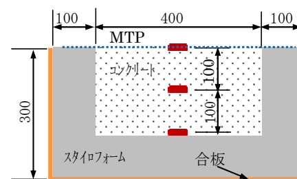
図2 保温効果確認用型枠
