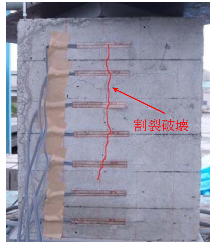
写真-1 割裂破壊状況
