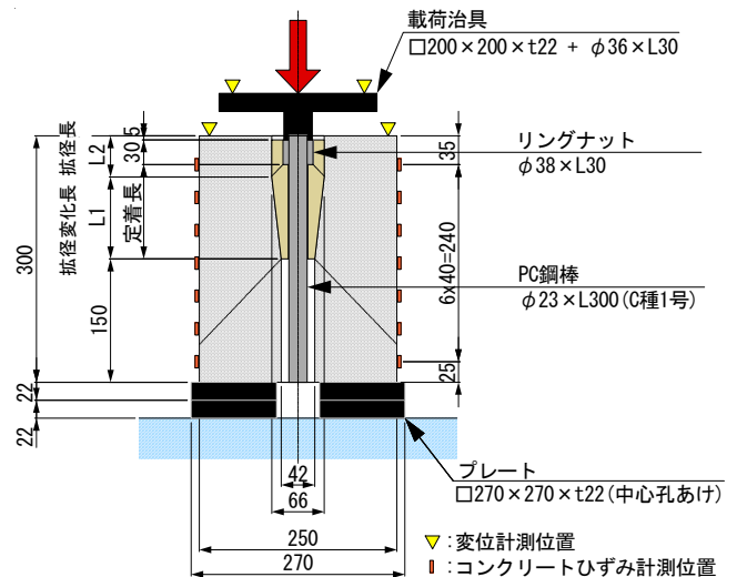
図-1 試験供試体の形状および載荷方法
