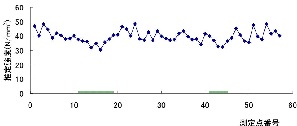
図3 推定強度測定値の変動
