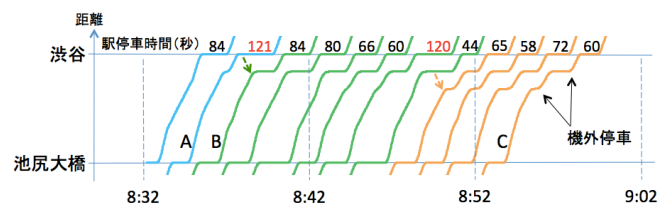
図5 余裕距離100mの距離—時間曲線
