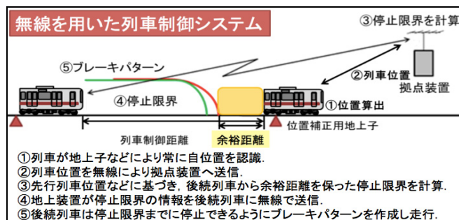
図 1 移動閉そくの仕組み
