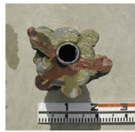
写真2 繰返し注入による補強体の造成例
