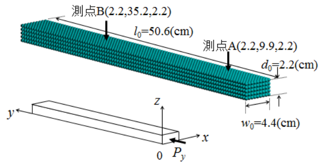
図-2 弾性波測定解析モデルと境界条件
