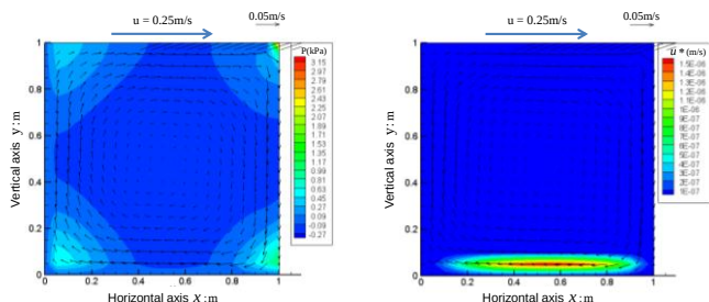
図3 圧力・流速分布
