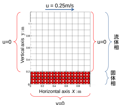
図5 連成解析条件
