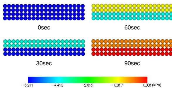
図7 固体相の間隙水圧分布
