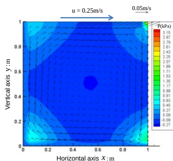
図2 流速・圧力分布
