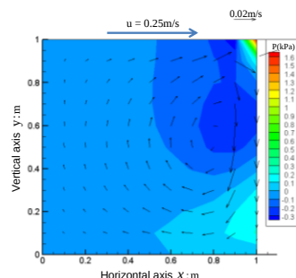
図6 流体相の流速・圧力分布
